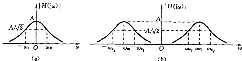
图 4-4 滤波器带宽
