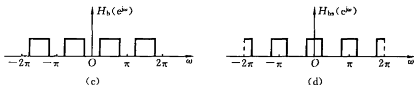
续图 5-1 理想频选滤波器的频率响应
