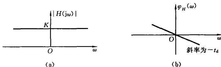
图 4-1 无失真传输系统的频率响应
