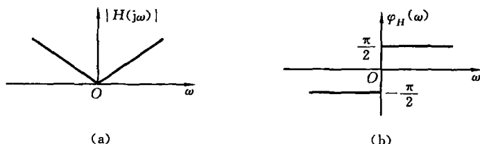
图 4-2 微分滤波器的频率响应
