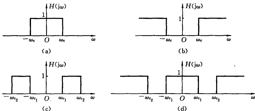
图 4-3 理想频率选择滤波器的频率响应
